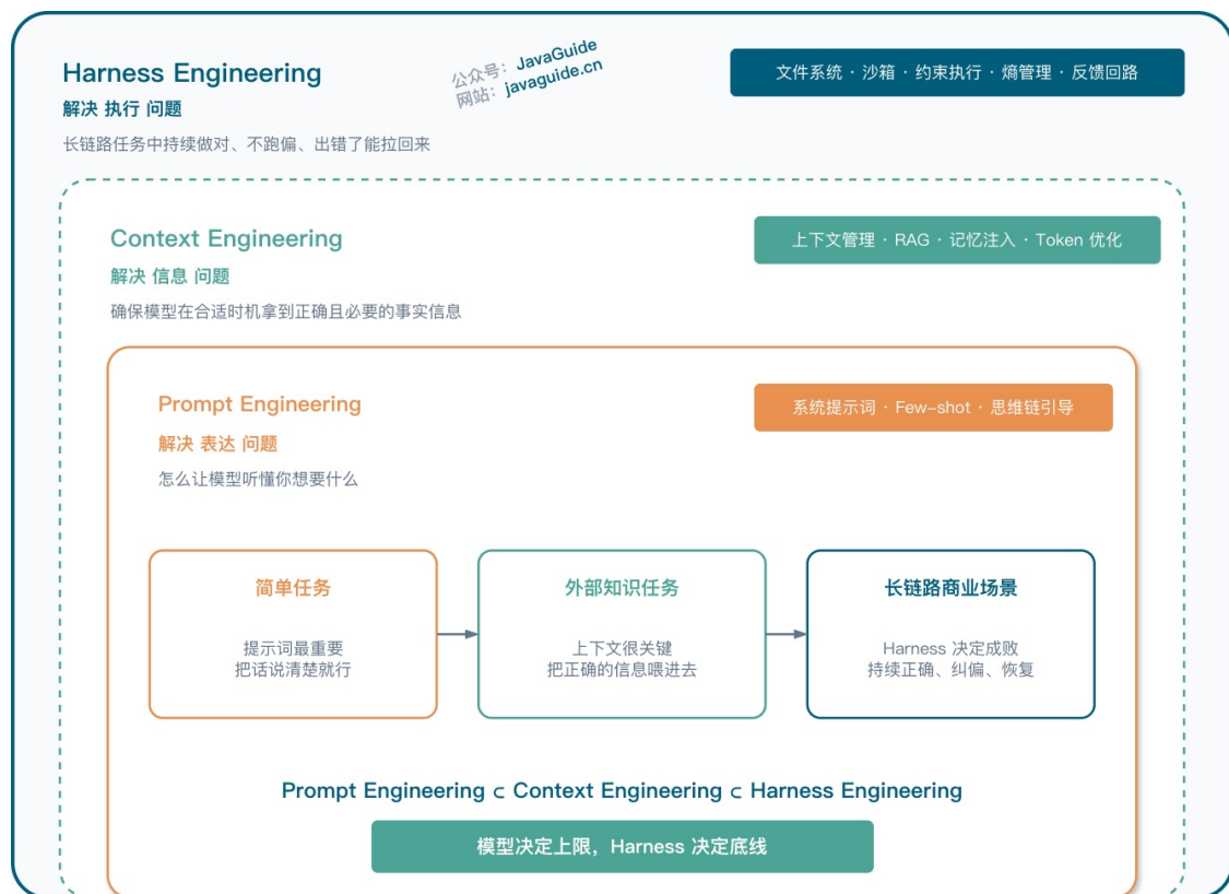
Harness 和 Prompt/Context Engineering 的关系
